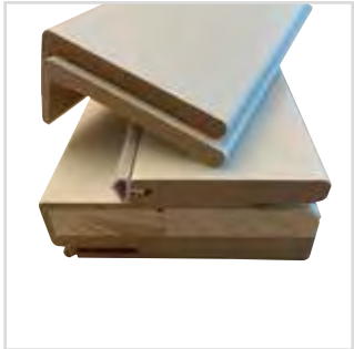
Stipite Sandwich con Coprifili MDF
